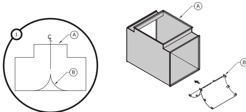
A: AMU tee B: Turning Vane Assembly
